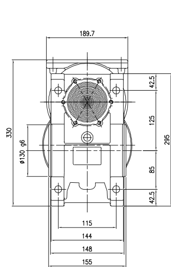
FLANGIA ATTACCO MOTORE GRANDEZZA 90 B14 (24/140)
